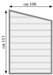
art. 520 Pannello Alto Inclinato Coibentato
