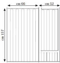
art. 500 Pannello Frontale con Cannello
